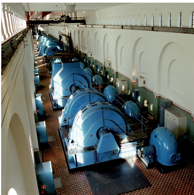
Turbinhall, Tyssedal kraftstasjon, Norsk Vasskraft og Industristadmuseum. Foto: Gunnbjørg Austrheim, HFK
