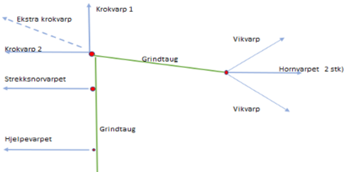
Figur 4 Varp-arrangement for enkelnot. Figur 4 viser typisk arrangement av varp for ei enkelnot som vist på figur 1. Lengden på streng/tau er ikke vist da denne varierte etter dybdeforhold (stor dybde=langt varp)
