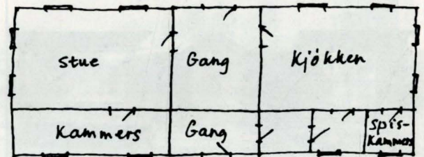
Hovedbygningen på Sandtrøen. Grunnplan 1. etasje. Bygningen har den vanlige planløsningen. Den er en variant av den såkalte midtkammersbygningen som har inngangsdøra og gangen på midten, et kammers bak gangen, og et stuerom i hver ende av huset.
