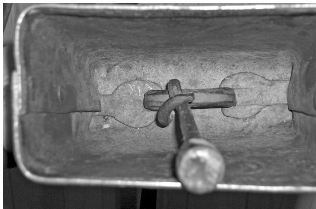
Dette er den måten Dalstrøsmedan' smidde fast bellhempa på, forma som eit rundt hjerte.
